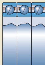
串联配置 代号后缀TT
