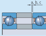
减少预载荷 (背对背)
