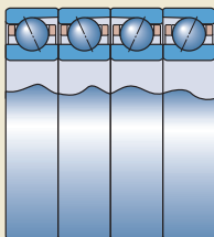
串联后面对面配置 代号后缀QFC
