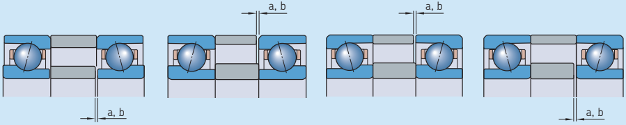
隔圈宽度减少量的指导值 - 719..E和70..E轴承系列
