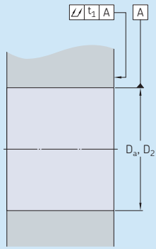
与螺栓安装和盒式轴承单元配合的轴承座的座孔和端面的几何精度
