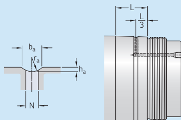
注油通道及配油槽的推荐尺寸
