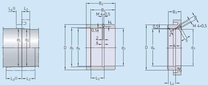
阶梯轴套及其安装面的推荐尺寸
