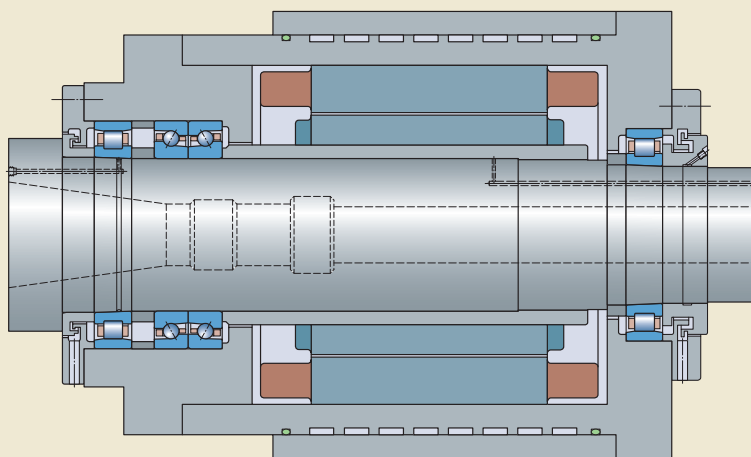
传统铣床主轴
