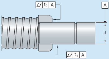
轴与轴承配合处的几何精度
