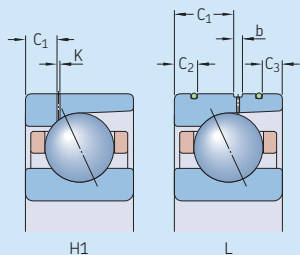
直接油气润滑的719..D和70..D轴承系列的外形尺寸
