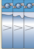
串联 代号后缀TT
