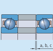
增加预载荷 (背对背)
