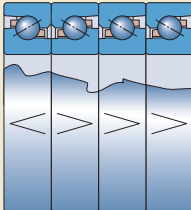
背对背串联 代号后缀QBT
