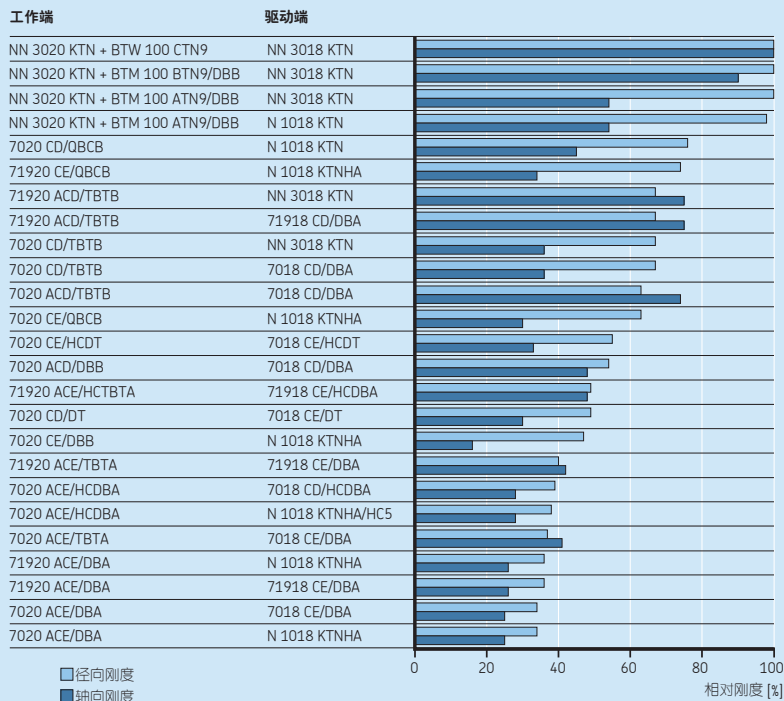
典型主轴轴承系统的相对刚度
