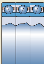
面对面+串联配置 代号后缀TFT
