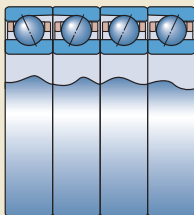
面对面+串联配置 代号后缀QFT
