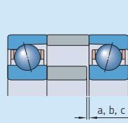
减少预载荷 (面对面)
