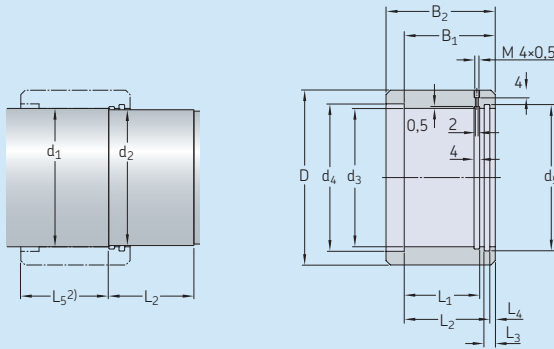
带O型圈的阶梯轴套及其安装面的推荐尺寸
