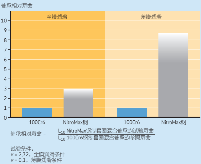
NitroMax钢制套圈混合陶瓷轴承的相对寿命
