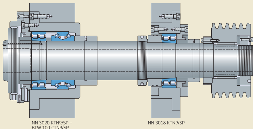
大直径棒料加工用的皮带驱动数控车床主轴
