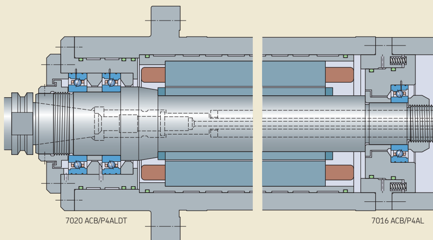
高速金属切削用电主轴
