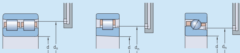
圆柱滚子轴承和双向推力角接触球轴承的喷油嘴位置
