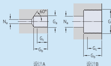
连接供油的螺纹孔的设计和推荐尺寸
