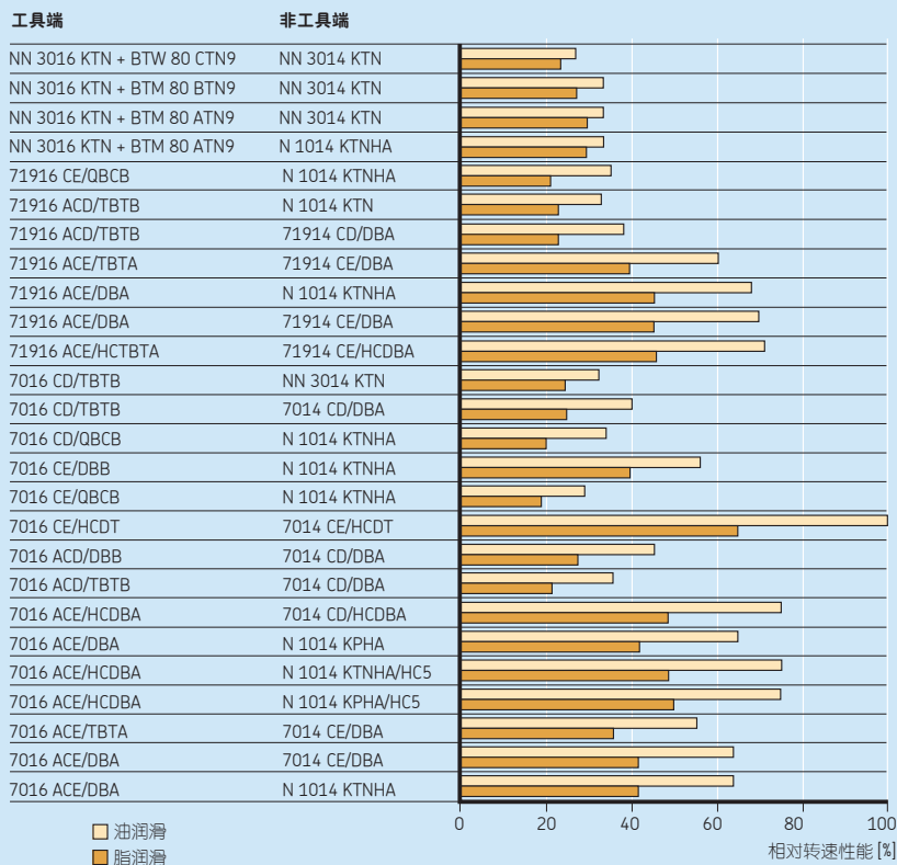
典型主轴轴承系统的相对转速性能
