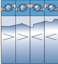
串联面对面 代号后缀QFC
