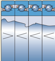
面对面串联 代号后缀QFT
