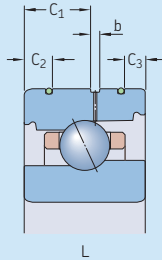
直接油气润滑的719..B和70..B轴承系列的外形尺寸
