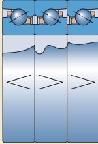
背对背串联 代号后缀TBT
