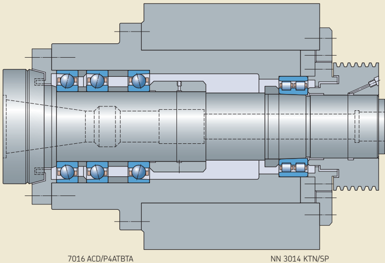
皮带驱动的数控车床主轴
