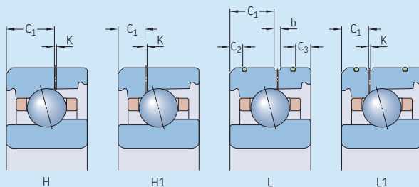
直接油气润滑的70..E轴承系列的外形尺寸
