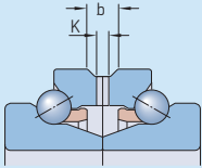
BTW..W33系列轴承环形槽和润滑孔的尺寸
