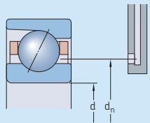
角接触球轴承喷嘴位置
