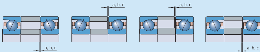
隔圈宽度减少量的指导值 - 719..D和70..D轴承系列
