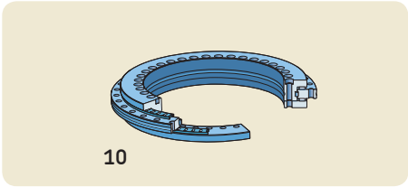
推力-向心圆柱滚子轴承 (→ 第319页) 基本设计 (NRT系列) (10)
