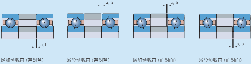
隔圈宽度减少量的指导值 - 718..D轴承系列
