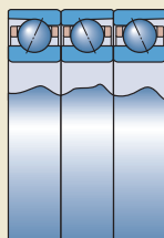
背对背+串联配置 代号后缀TBT
