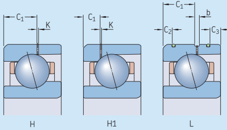
直接油气润滑的719..E轴承系列的外形尺寸
