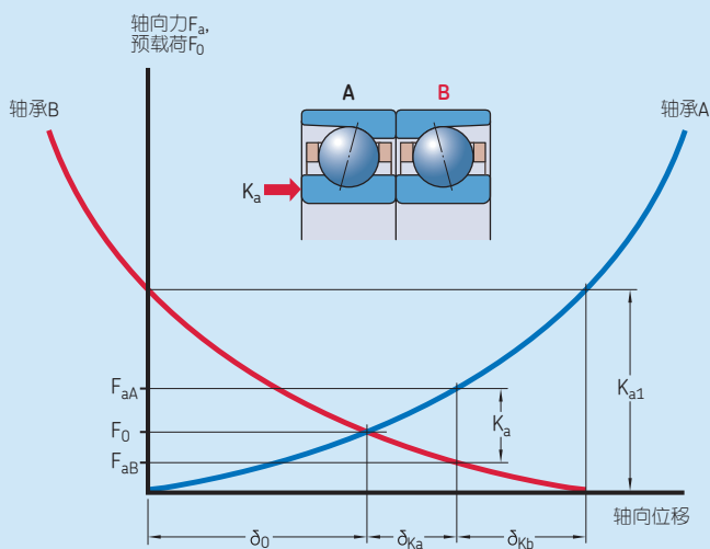
外部载荷对已施加预载荷的轴承组的影响
