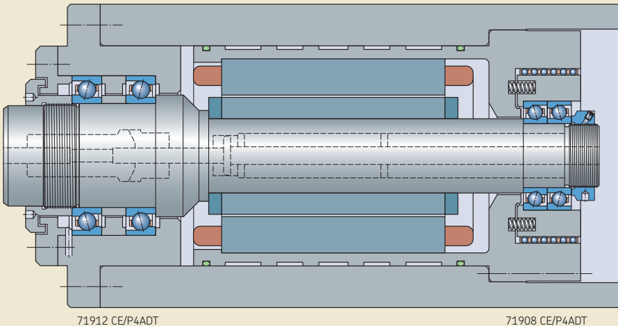
内圆磨床用电主轴
