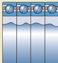
串联配置 代号后缀QT
