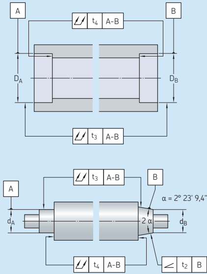
轴上及轴承座中轴承安装面的形位公差
